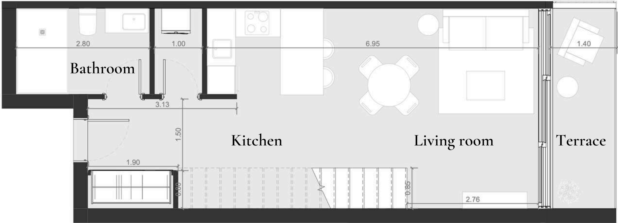
PLANTA PRIMERA
